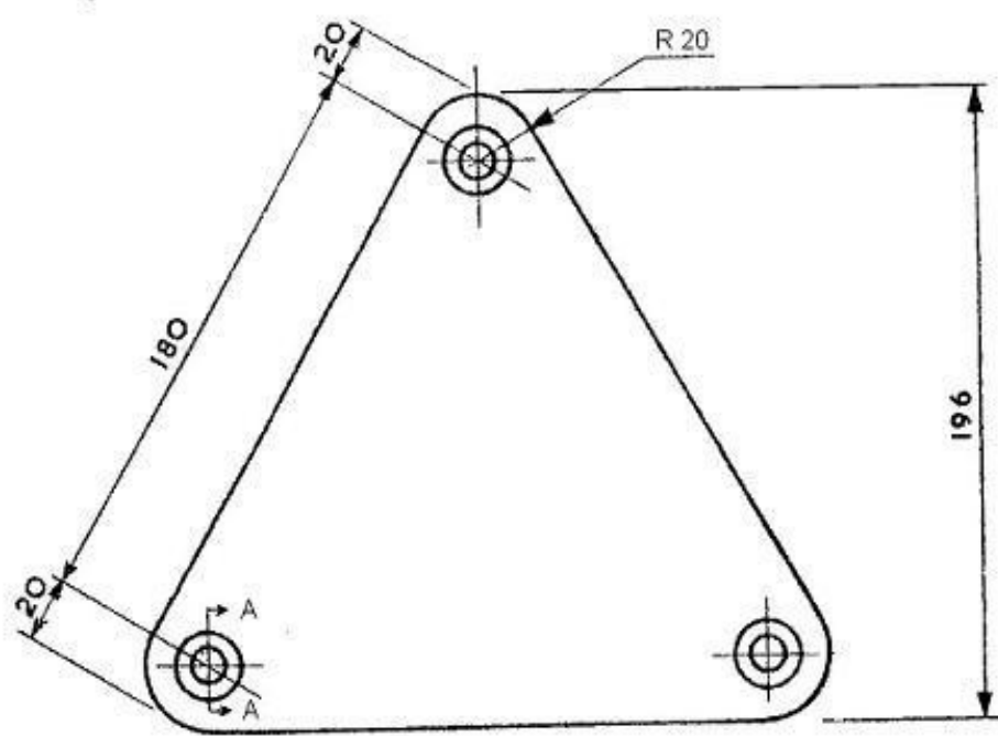
Τρίποδο ηλεκτρόδιο
