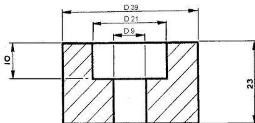
Κυλινδρικό πόδι ηλεκτροδίου Τομή Α- Α
